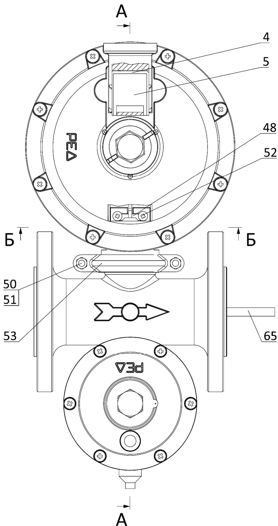
Рисунок 1 – Устройство регулятора давления «РЕД-3-40-Н-...».
