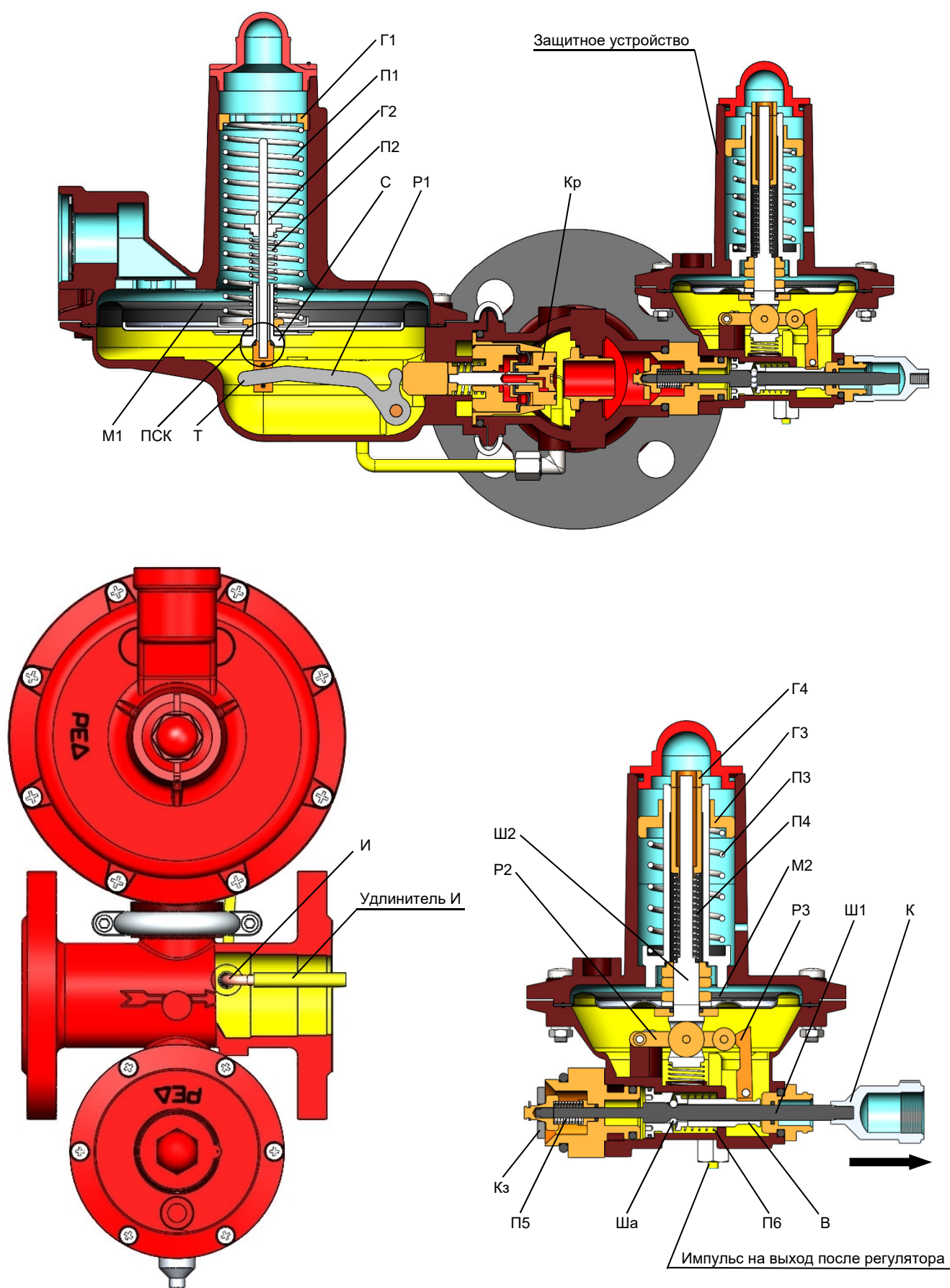
Рисунок 1 – Конструкция регуляторов давления «РЕД-3-40».
