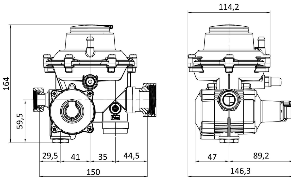
Рисунок 3 – Габаритные размеры регуляторов давления «РЕД-1»
